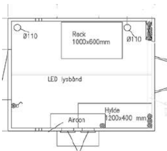
Serverrum med aircondition, serverrack og indgangsdør med kodelås
